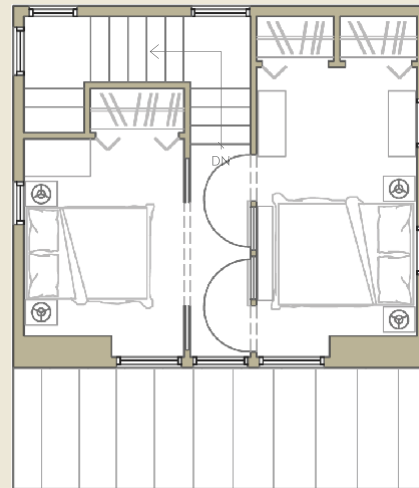
U P P E R L E V E L 3 1 5 S F
