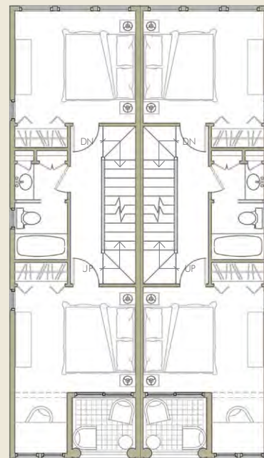
UPPER LEVEL 490 SF
