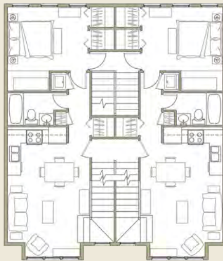
U P P E R L E V E L S 1,854 SF
